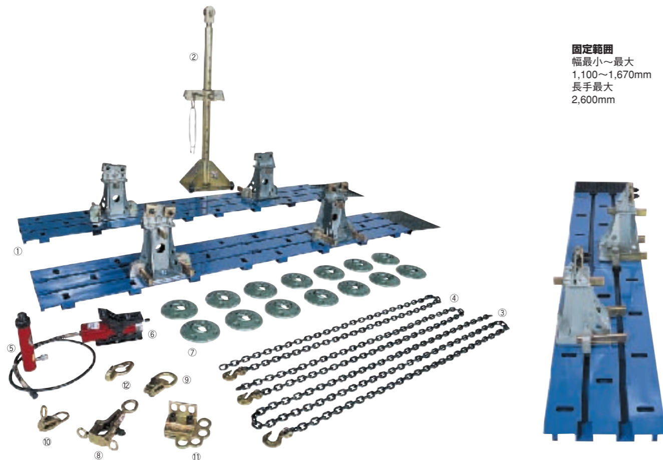
設置の一例 (単位/mm)
